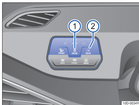
图 68 仪表盘局部视图：灯光按钮
