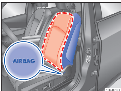
图 30 前排座椅侧面：侧面安全气囊的安装位置和膨胀范围
