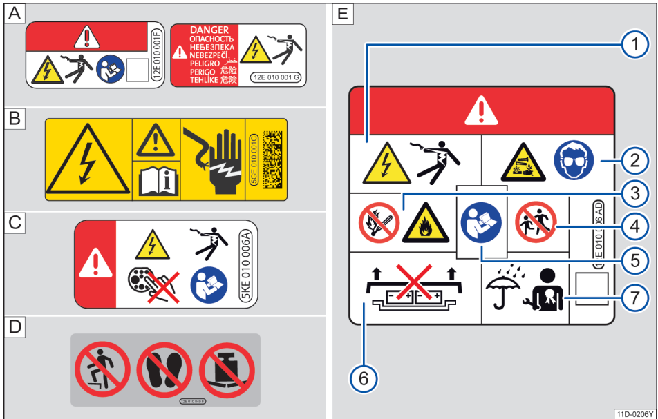
图 114 车型警告牌（示意图）：A. 高压组件 B. 高电压普通警告牌 C. 充电口高压警示标签 D、E. 高压电池上的警告牌
