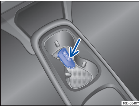
图 83 在中控台中：应急启动功能
